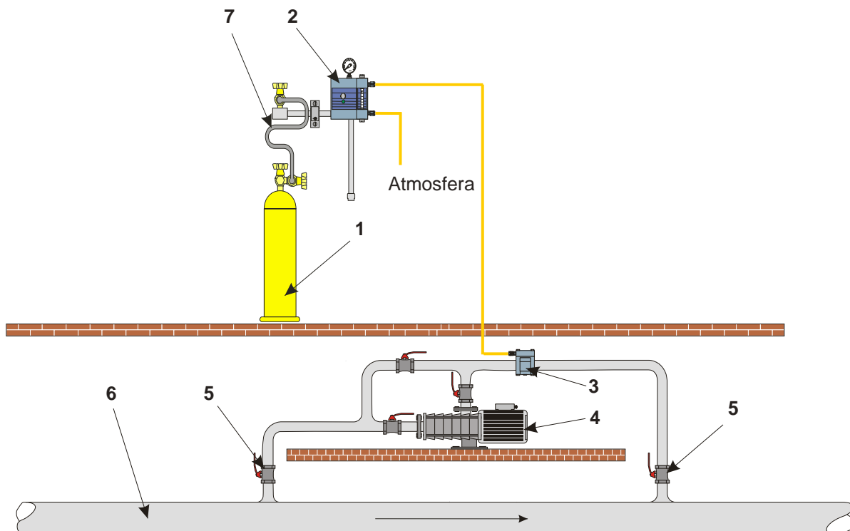
SISTEM DE CLORINARE CU CLOR GAZOS - DC 2.1 - tc
